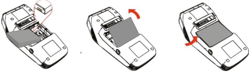
Şekil 4.3. Bataryanın Takılması
