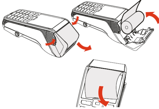
Şekil 4.5. Yazarkasaya Kağıt Takılması
