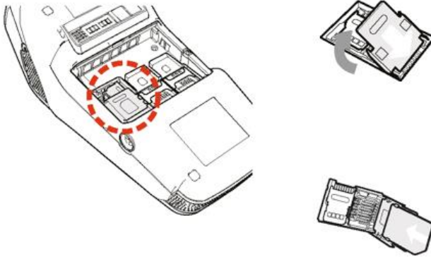
Şekil 4.1. Yazarkasa SIM Kartının Takılması
