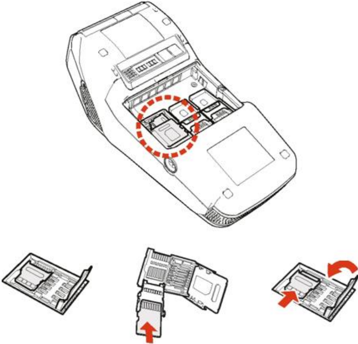
Şekil 4.2. Micro SD Kartın Takılması
